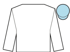
CUMULONIMBUS
